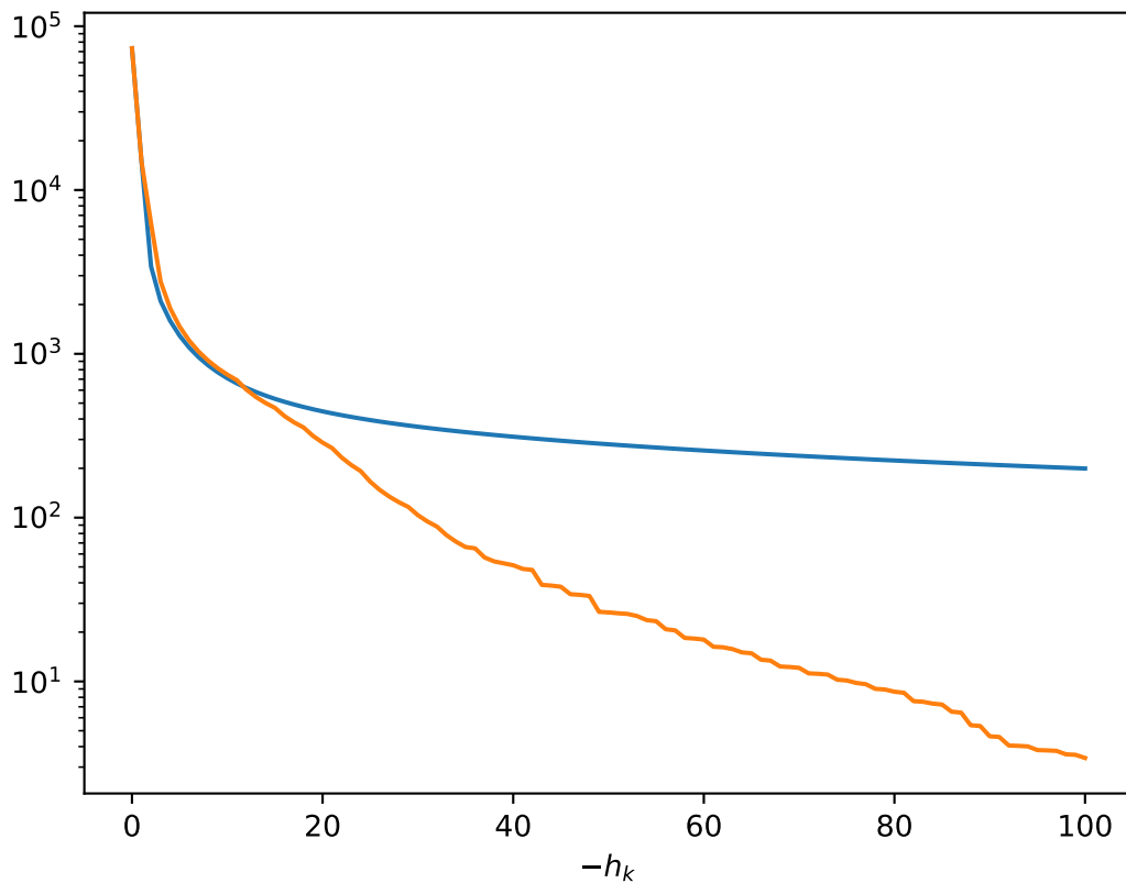
Gráfica de los métodos, iteraciones (k) vs -h_k
